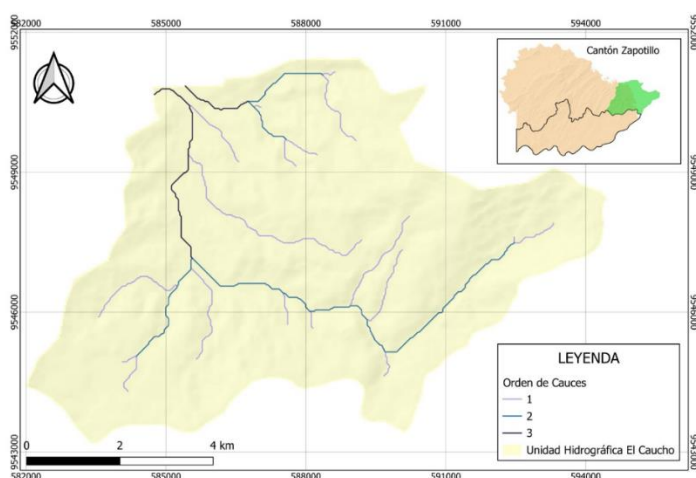
Figura 7. Distribución espacial de los cauces en la Unidad Hidrográfica El Caucho.
