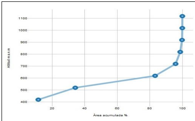
Figura 4. Curva Hipsométrica Unidad Hidrográfica Cazaderos.
