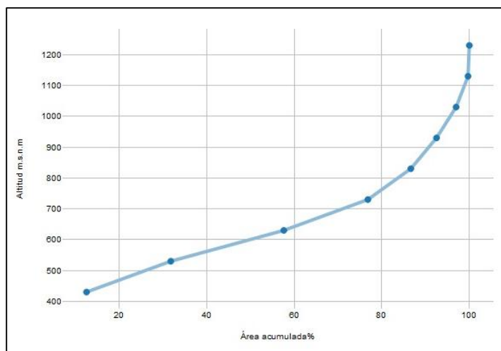
Figura 6. Curva hipsométrica de la Unidad Hidrográfica El Caucho.
