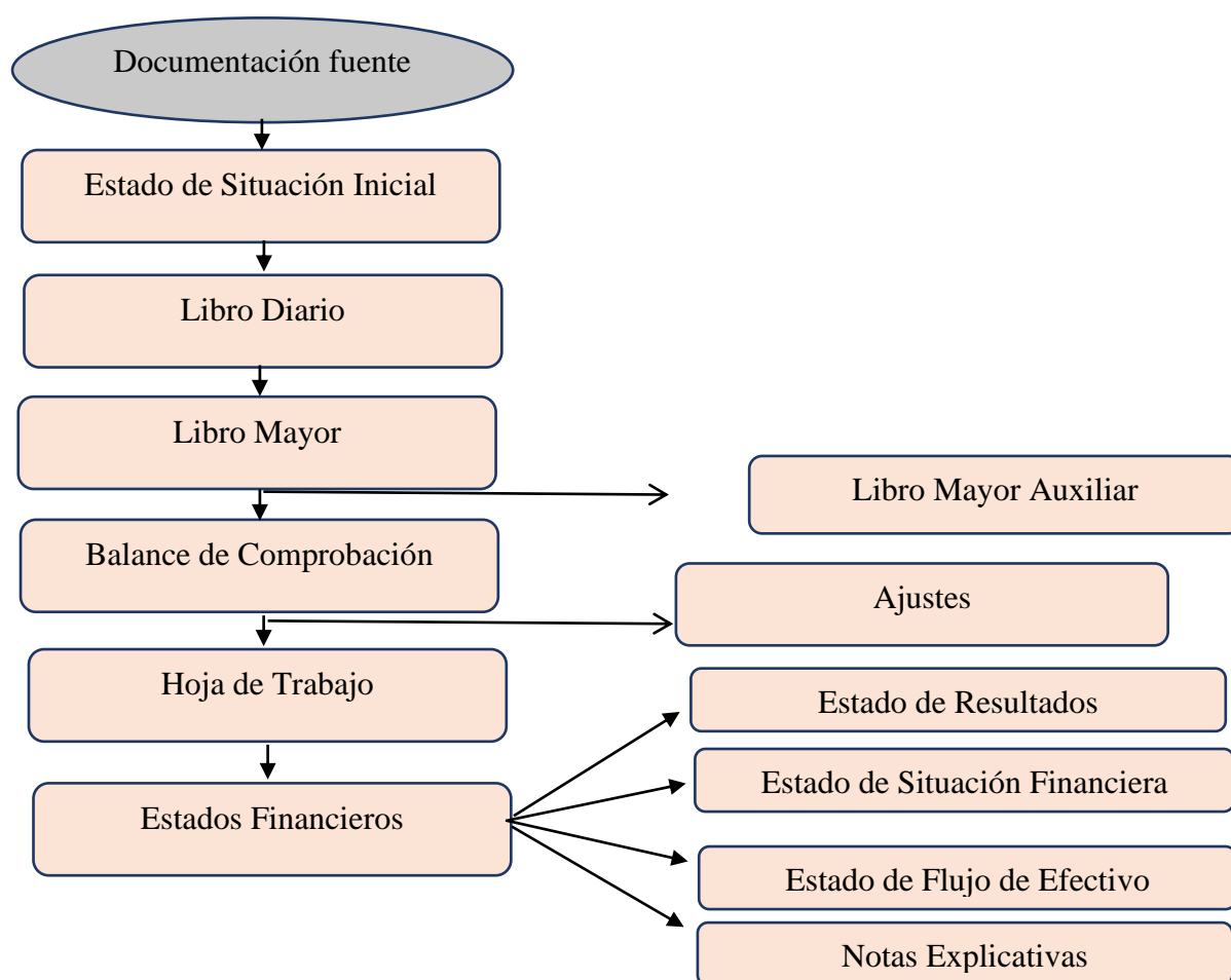
Figura 2. Estructura del proceso contable
