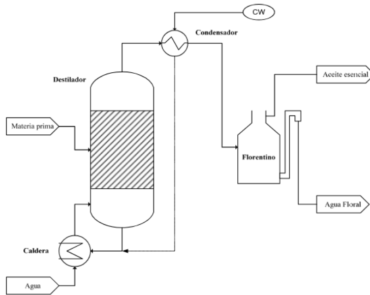
Figura 8. Esquema básico del proceso de extracción del aceite esencial por arrastre de vapor de agua (Cerpa, 2007).
