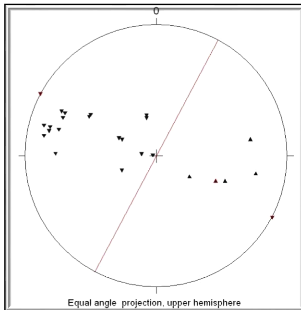
Figura 14. Representación estereográfica de las foliaciones.
