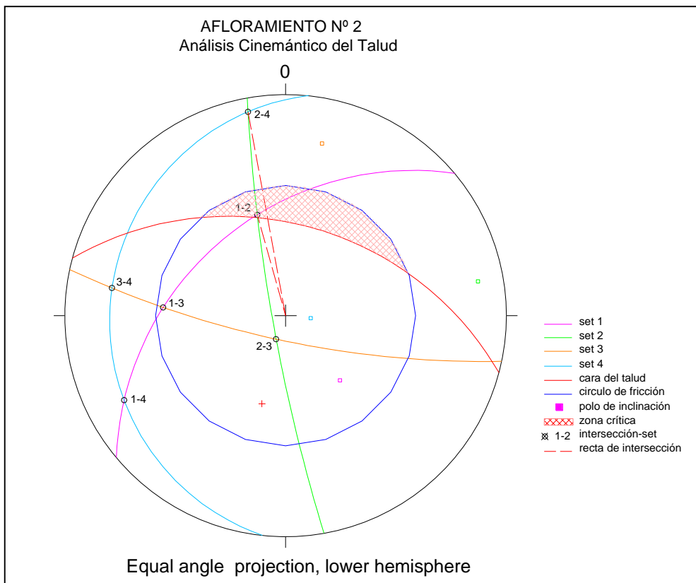
Figura 30. Análisis Cinemático del Afloramiento n 2
