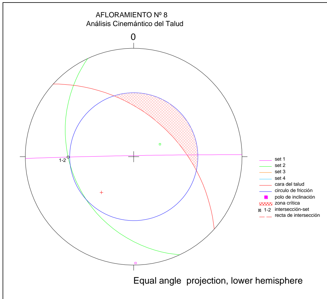
Figura 36. Análisis Cinemático del Afloramiento n 8
