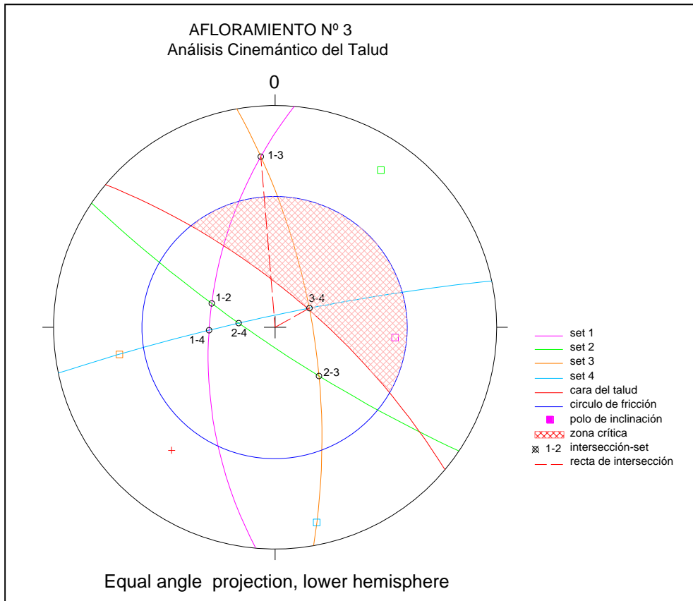
Figura 31. Análisis Cinemático del Afloramiento n 3
