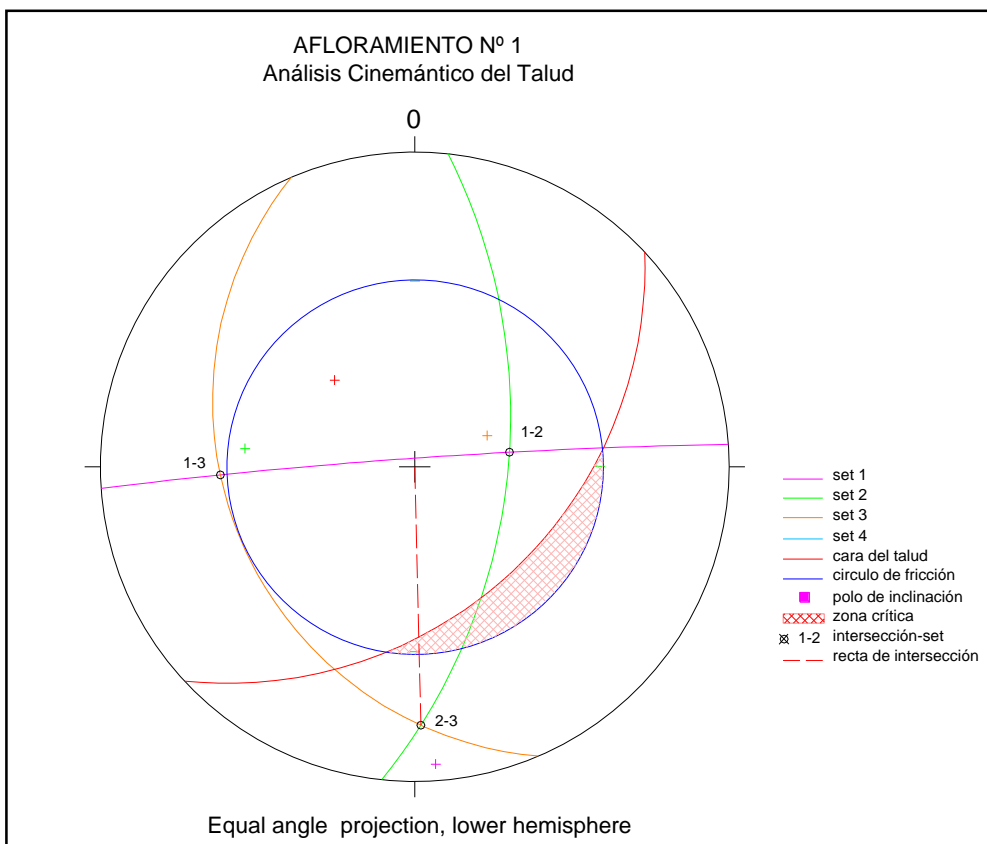
Figura 29. Análisis Cinemático del Afloramiento n 1
