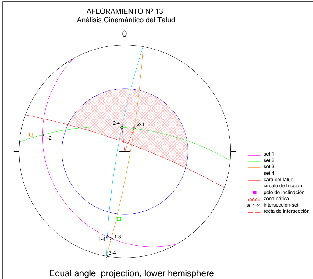
Figura 38. Análisis Cinemático del Afloramiento n 13
