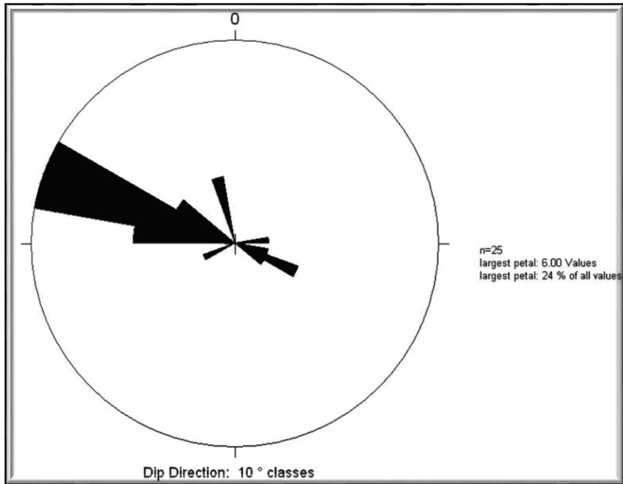
Figura 13. Diagrama de la rosa representando la foliación del macizo rocoso.
