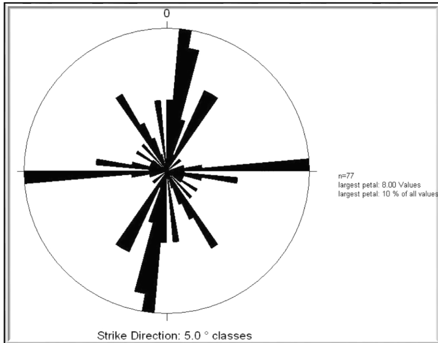
Figura 15. Diagrama de la rosa representado la dirección o rumbo de las diaclasas
