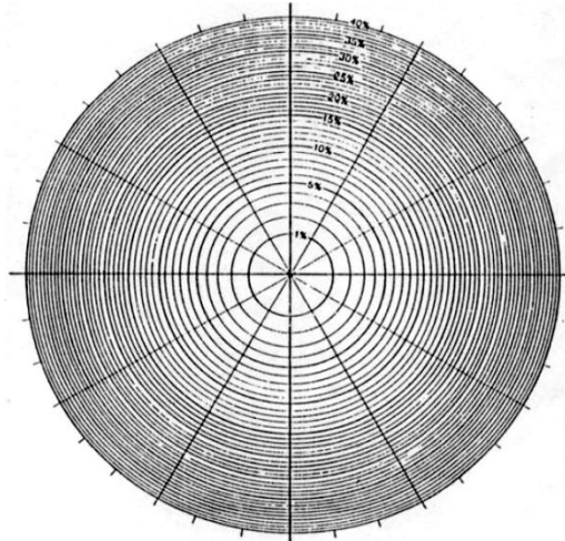
Figura 2. Diagrama de la Rosa.
