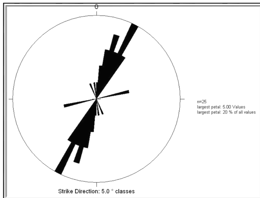
Figura 12. Diagrama de la rosa representando la dirección o rumbo del macizo rocoso
