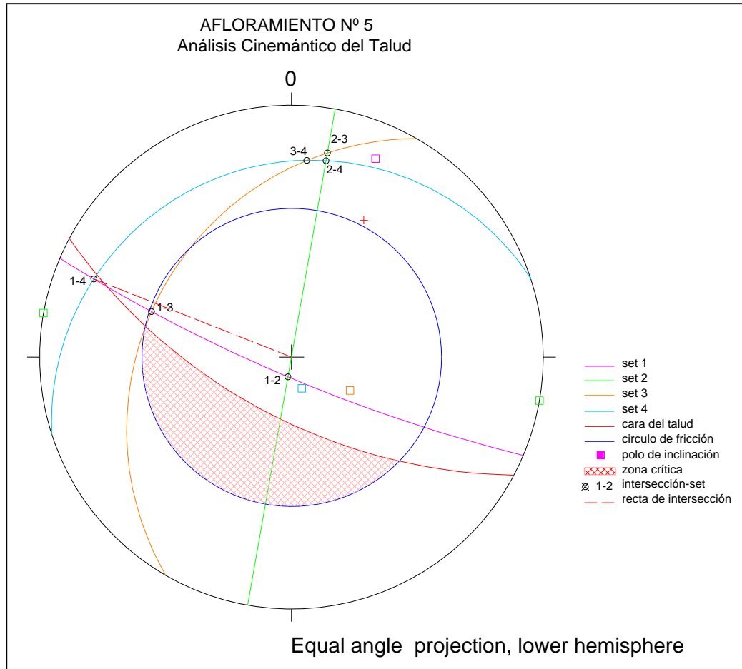
Figura 33 Análisis Cinemático del Afloramiento n 5
