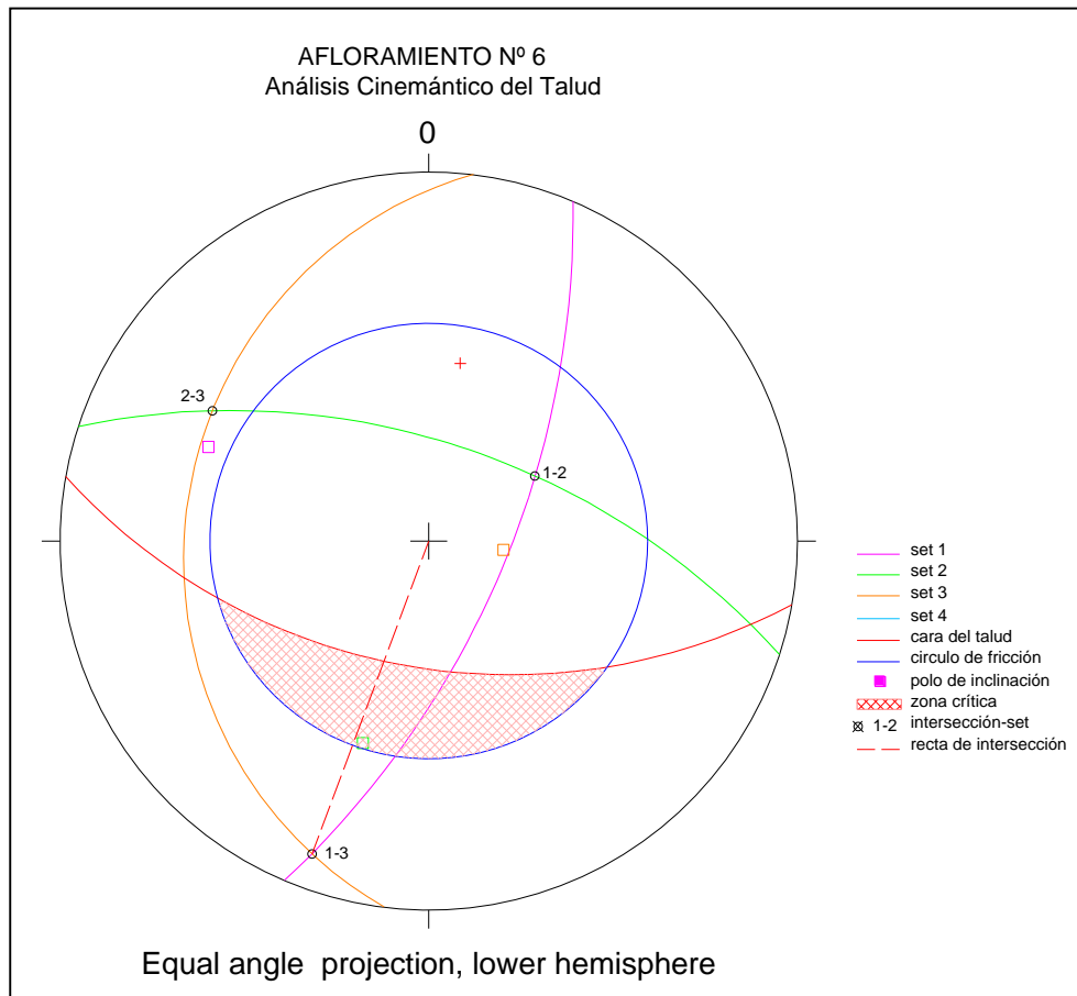
Figura 34 Análisis Cinemático del Afloramiento n 6
