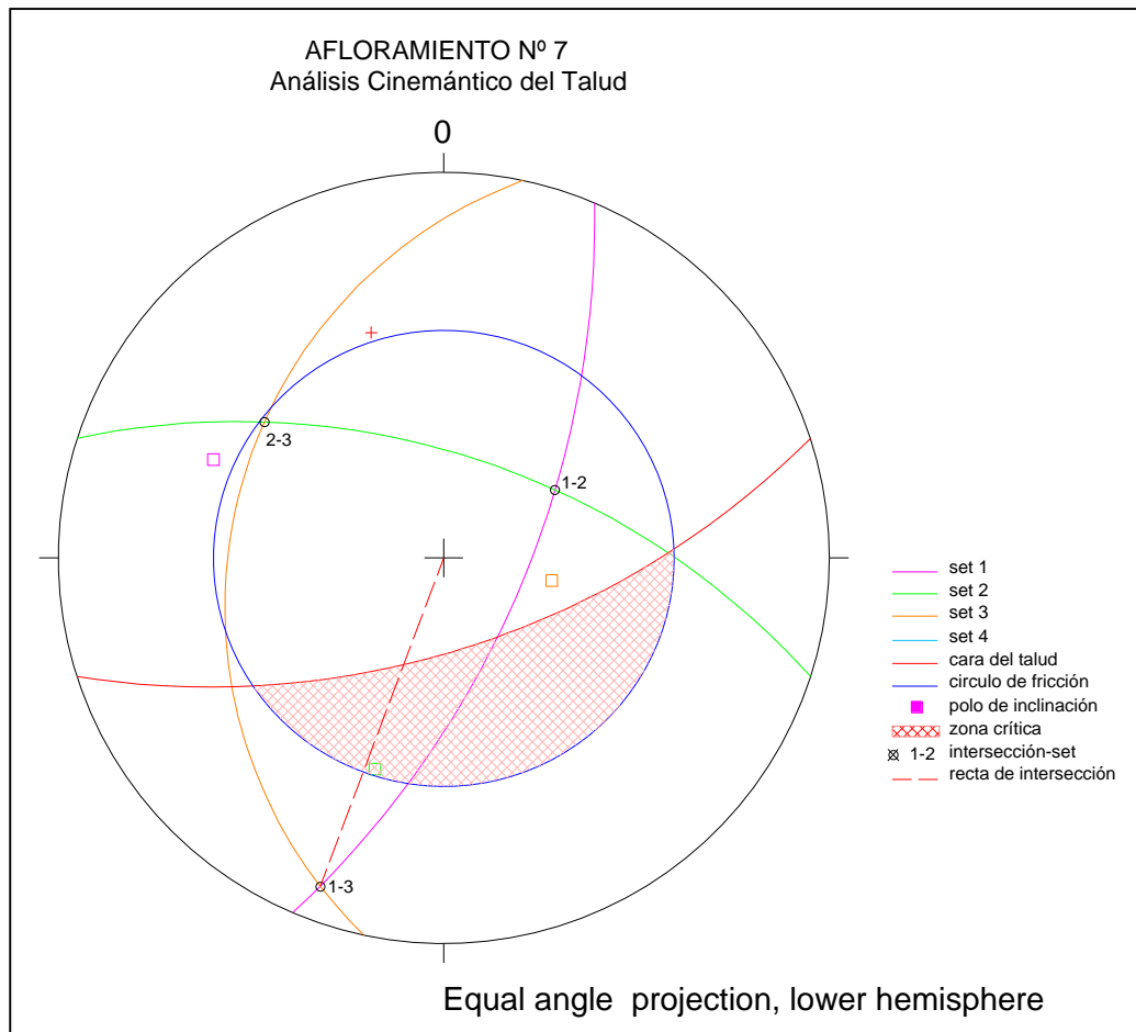
Figura 35. Análisis Cinemático del Afloramiento n 7
