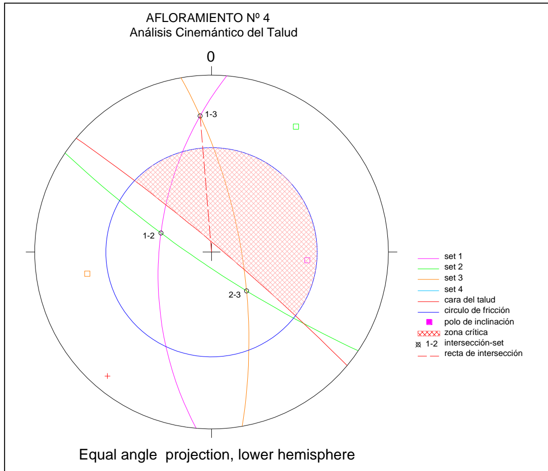
Figura 32. Análisis Cinemático del Afloramiento n 4
