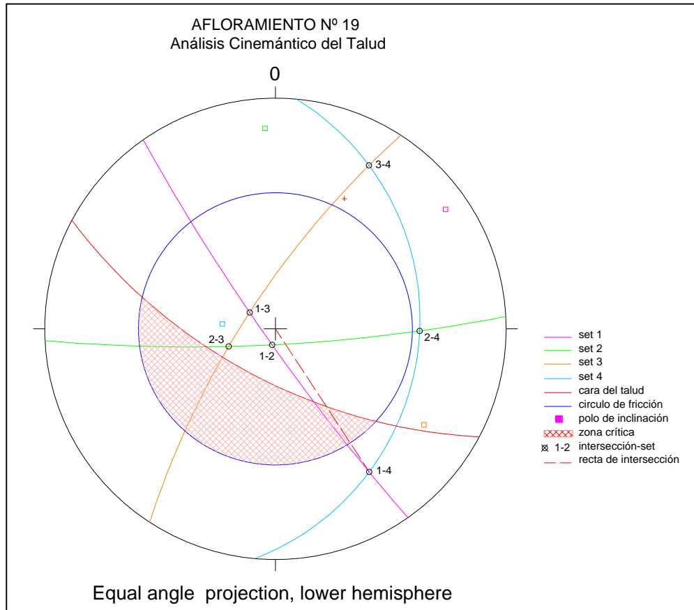
Figura 41. Análisis Cinemático del Afloramiento n 19
