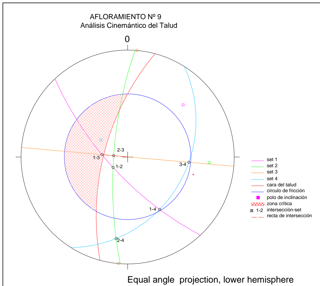
Figura 37. Análisis Cinemático del Afloramiento n 9
