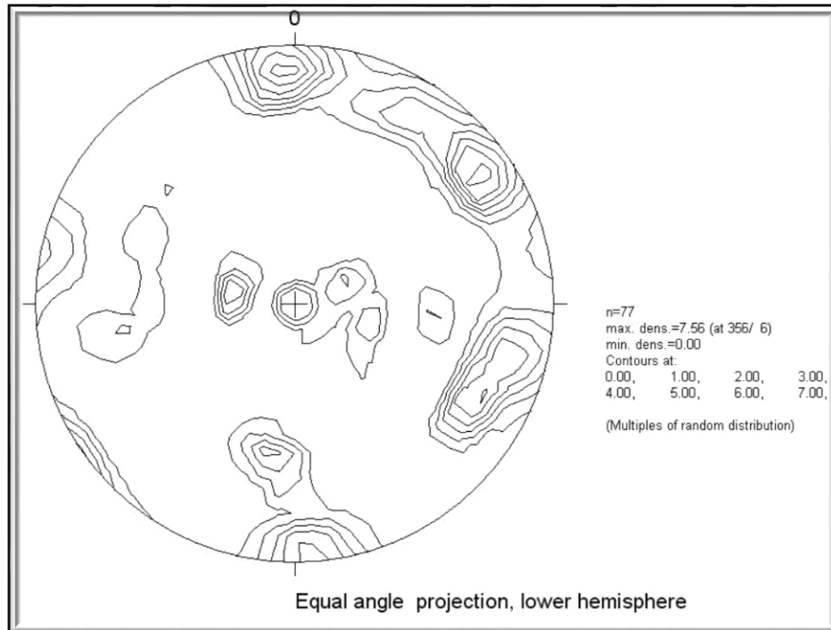
Figura 17. Representación de Diaclasas en la Red Estereográfica Polar
