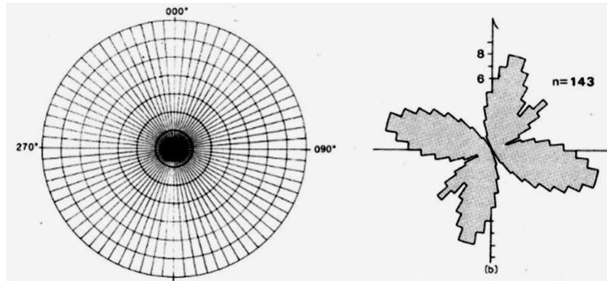
Figura 3. Diagramas de Rosa a) Diagrama que es usado para representar diagramas de la Rosa b) Diagramas de rosa completado con 143 mediciones.
