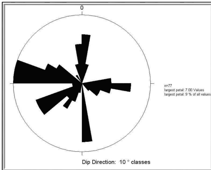
Figura 16. Diagrama de la rosa representando la inclinación de las diaclasas
