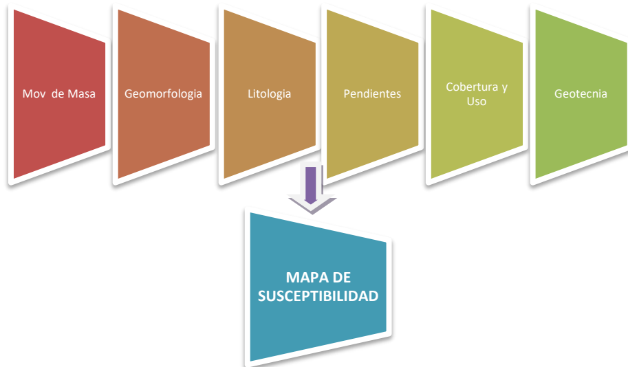
.Figura 42. Uso de SIG para combinación de mapas
