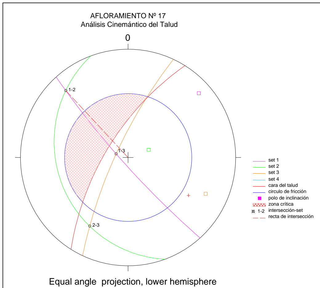
Figura 39. Análisis Cinemático del Afloramiento n 17
