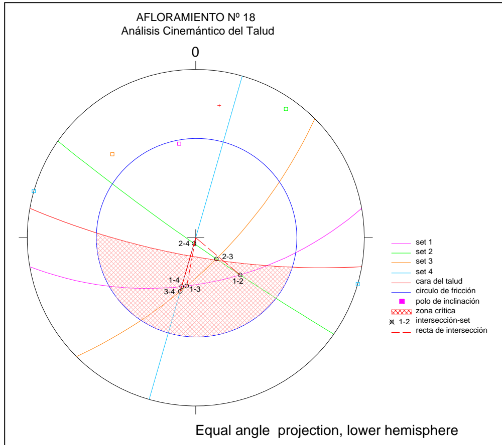
Figura 40. Análisis Cinemático del Afloramiento n 18
